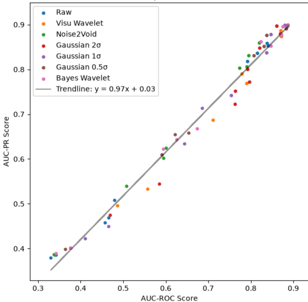
AUC Scatterplot (Dataset View)
